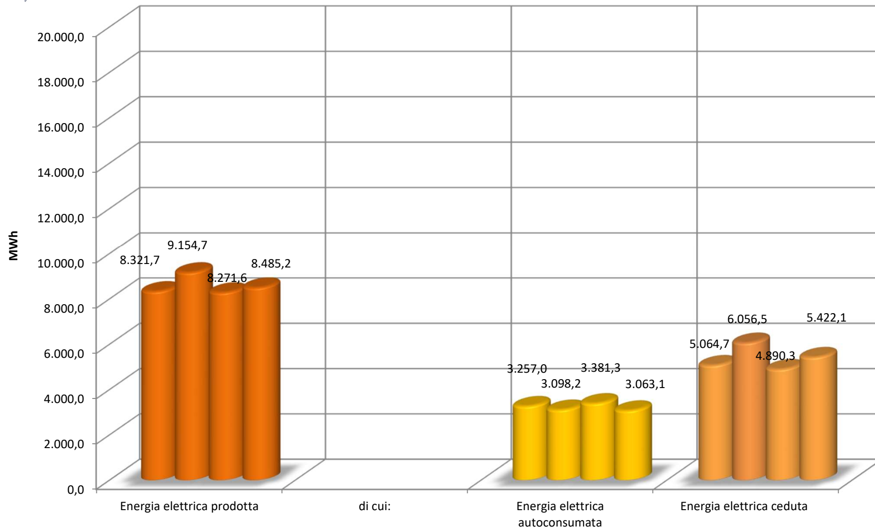
Grafico_Energia elettrica_25
