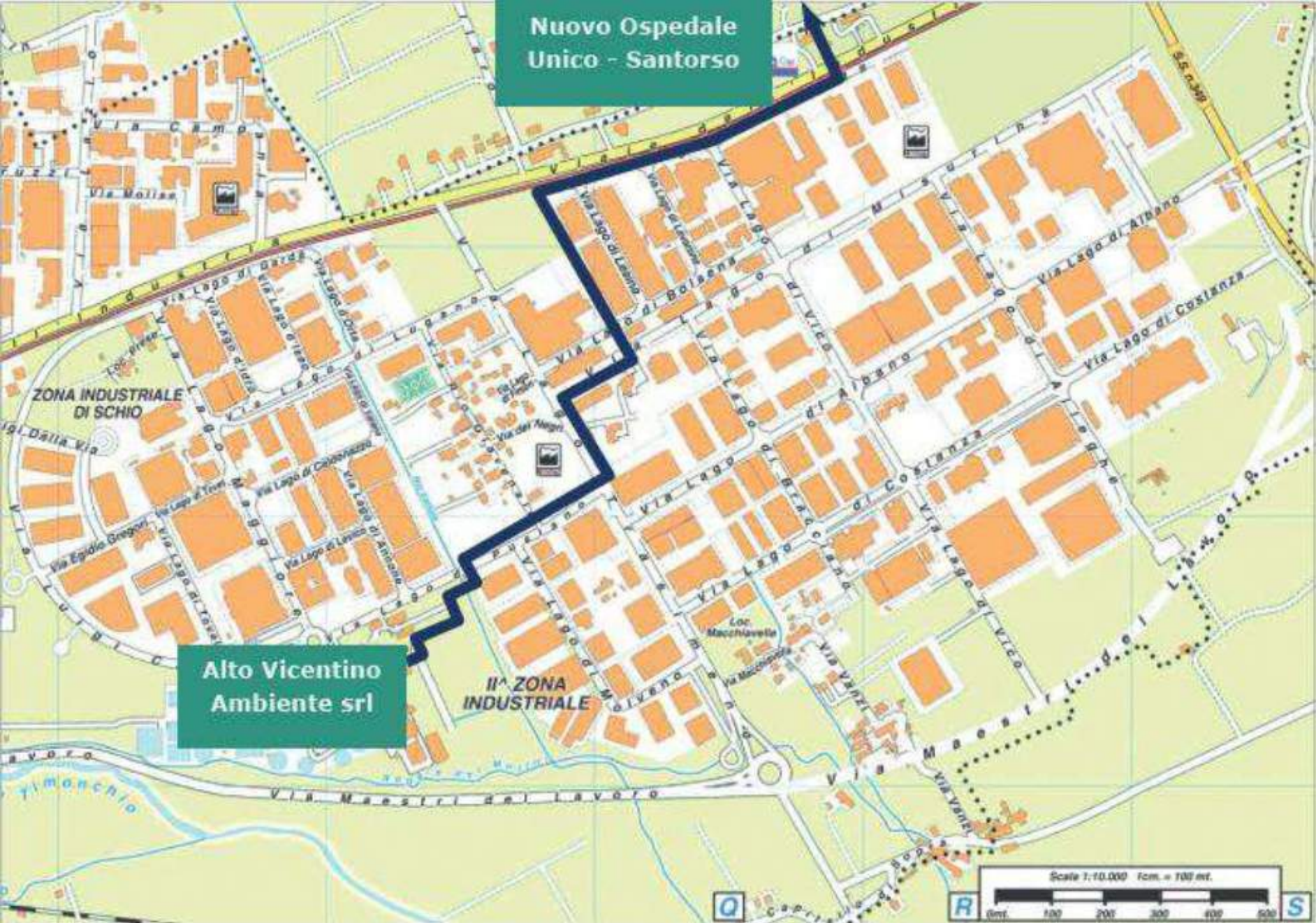
In blu il percorso delle tubazioni della rete di teleriscaldamento che collegano Alto Vicentino Ambiente (Schio) al nuovo polo ospedaliero dell'Alto Vicentino (Santorso),
